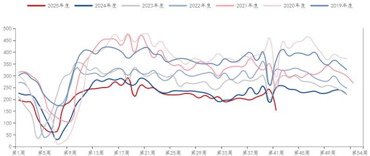
图 6：表观需求量 螺纹钢：消费量：中国（周）
