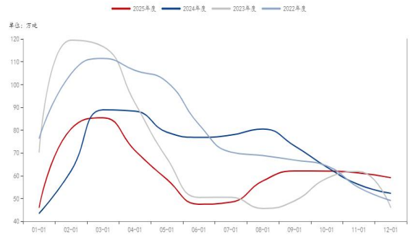
图 18：2022-2025 年电解铝现货库存
