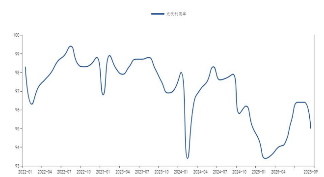
图 16：光伏利用率
