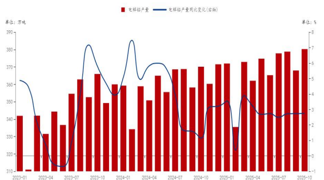
图 6：电解铝产量
